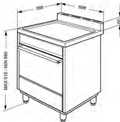
DESENHO TÉCNICO Nº 70
