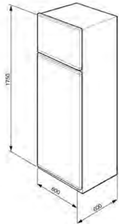
DESENHO TÉCNICO Nº 158
