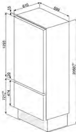
DESENHO TÉCNICO Nº 133
