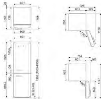
DESENHO TÉCNICO Nº 138
