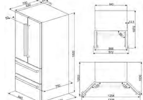
DESENHO TÉCNICO Nº 150
