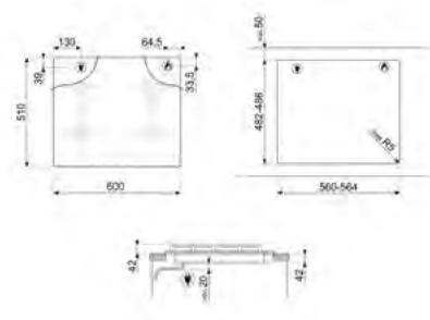
DESENHO TÉCNICO Nº 53
