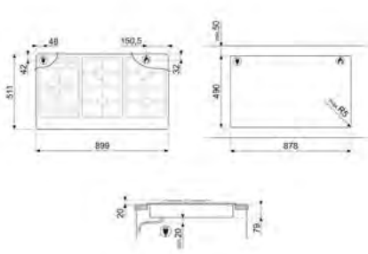
DESENHO TÉCNICO Nº 44
