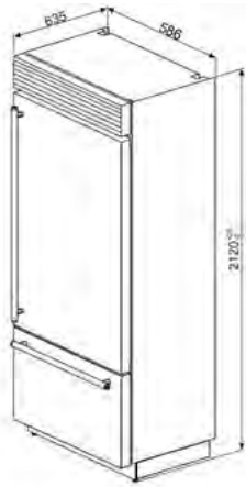
DESENHO TÉCNICO Nº 130
