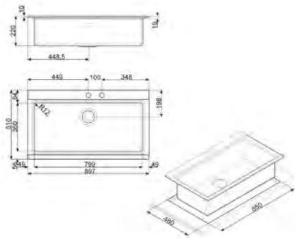
DESENHO TÉCNICO Nº 191
