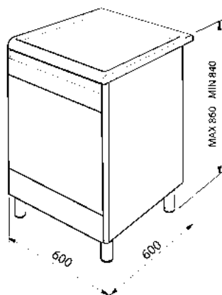
DESENHO TÉCNICO Nº 76
