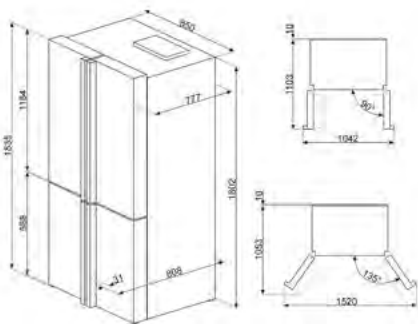
DESENHO TÉCNICO Nº 148
