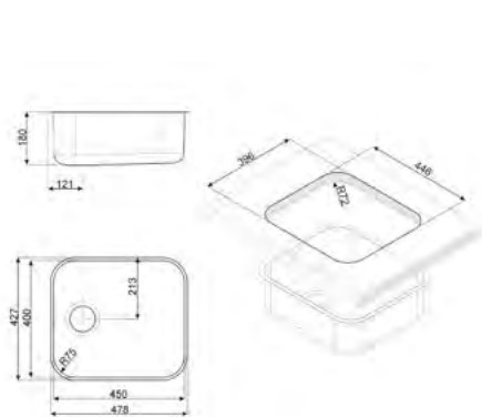
DESENHO TÉCNICO Nº 206
