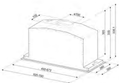
DESENHO TÉCNICO Nº 123
