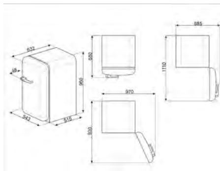
DESENHO TÉCNICO Nº 141
