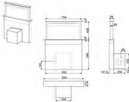
DESENHO TÉCNICO Nº 80
