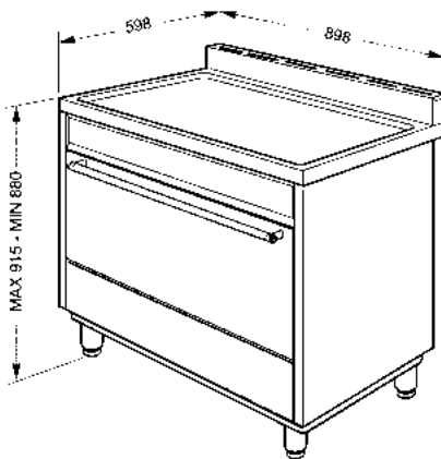
DESENHO TÉCNICO Nº 69
