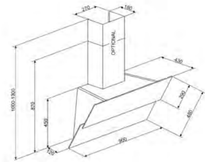
DESENHO TÉCNICO Nº 94
