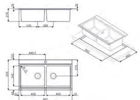
DESENHO TÉCNICO Nº 208
