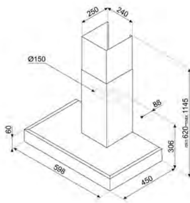
DESENHO TÉCNICO Nº 113
