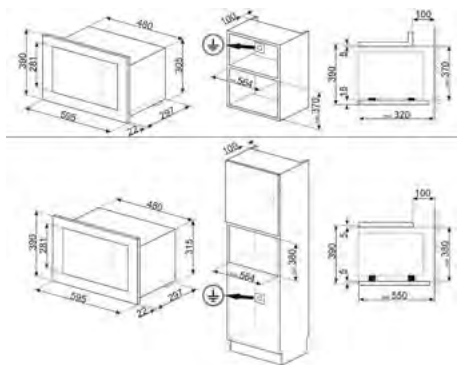
DESENHO TÉCNICO Nº 10
