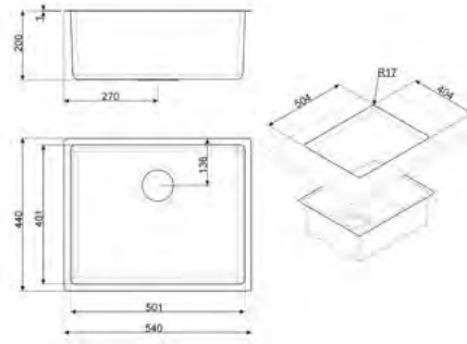
DESENHO TÉCNICO Nº 201
