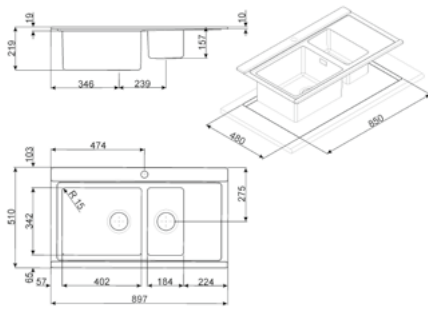
DESENHO TÉCNICO Nº 209
