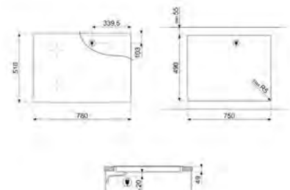
DESENHO TÉCNICO Nº 26
