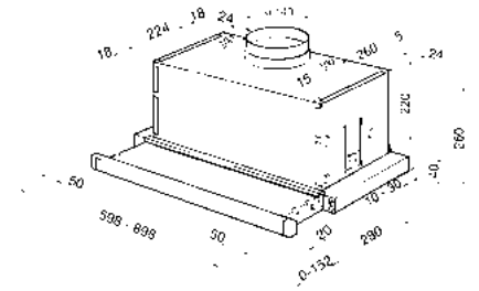
DESENHO TÉCNICO Nº 128
