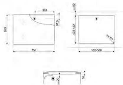
DESENHO TÉCNICO Nº 27
