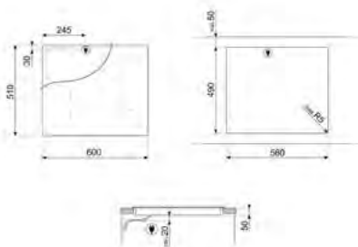
DESENHO TÉCNICO N° 35
