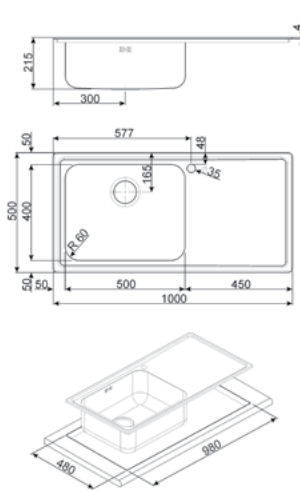
DESENHO TÉCNICO Nº 216
