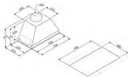
DESENHO TÉCNICO Nº 120
