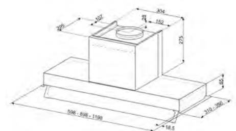
DESENHO TÉCNICO Nº 117
