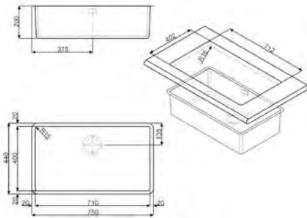
DESENHO TÉCNICO Nº 200
