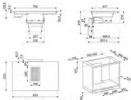
DESENHO TÉCNICO Nº 16
