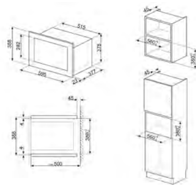
DESENHO TÉCNICO Nº 8
