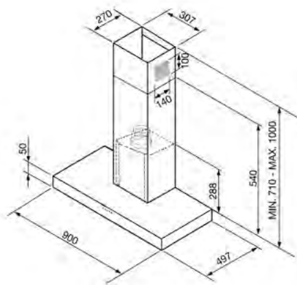
DESENHO TÉCNICO Nº 109
