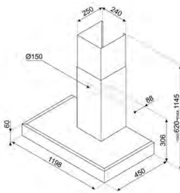
DESENHO TÉCNICO Nº 110
