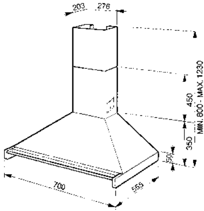
DESENHO TÉCNICO Nº 103
