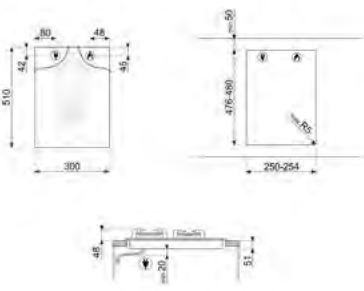
DESENHO TÉCNICO Nº 59
