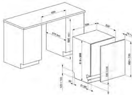
DESENHO TÉCNICO Nº 177
