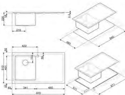
DESENHO TÉCNICO Nº 213
