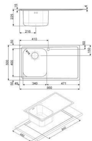
DESENHO TÉCNICO Nº 217
