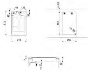
DESENHO TÉCNICO Nº 55
