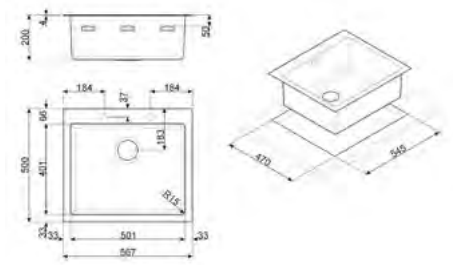
DESENHO TÉCNICO Nº 193
