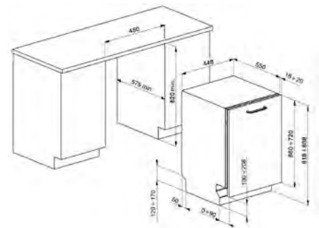
DESENHO TÉCNICO Nº 181
