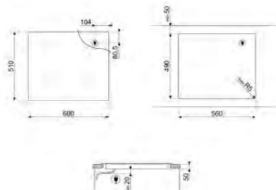
DESENHO TÉCNICO Nº 22
