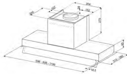
DESENHO TÉCNICO Nº 119
