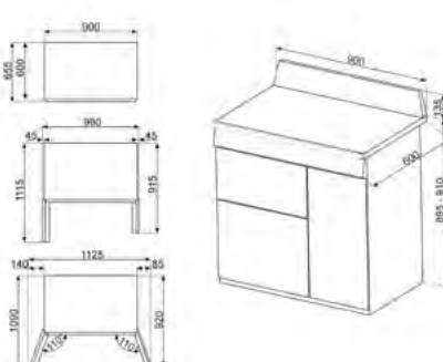
DESENHO TÉCNICO Nº 66
