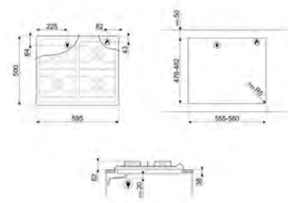
DESENHO TÉCNICO Nº 52
