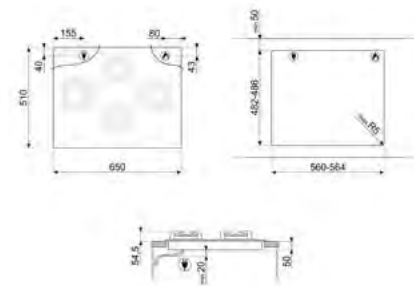
DESENHO TÉCNICO Nº 41
