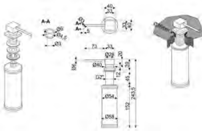
DESENHO TÉCNICO Nº 230
