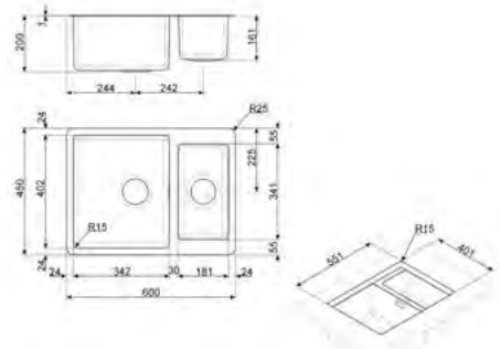
DESENHO TÉCNICO Nº 199
