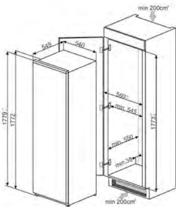
DESENHO TÉCNICO Nº 162
