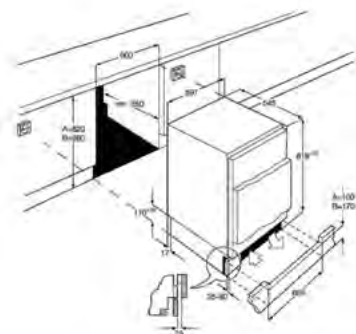
DESENHO TÉCNICO Nº 166
