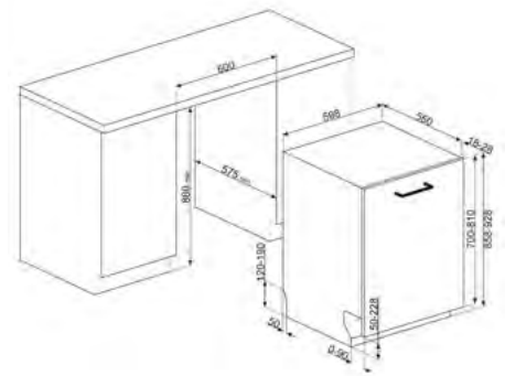
DESENHO TÉCNICO Nº 178
