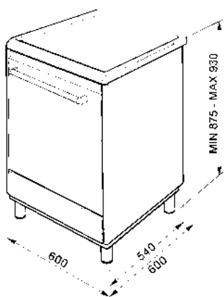
DESENHO TÉCNICO Nº 78
