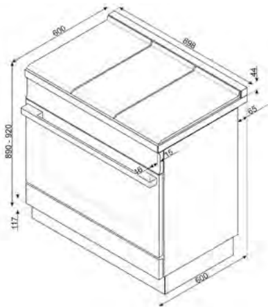
DESENHO TÉCNICO Nº 68
