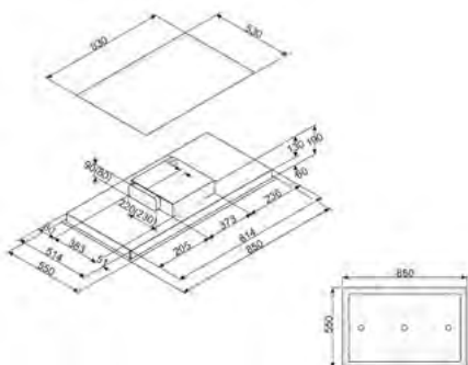
DESENHO TÉCNICO Nº 86
