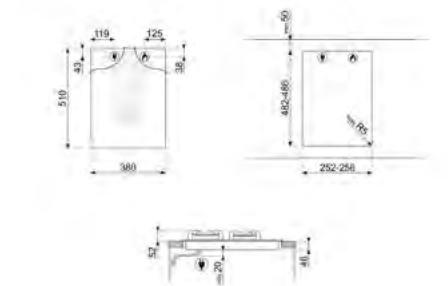
DESENHO TÉCNICO Nº 42
