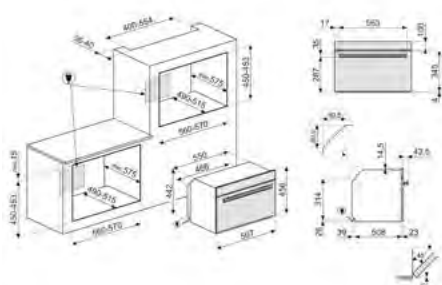
DESENHO TÉCNICO Nº 5
