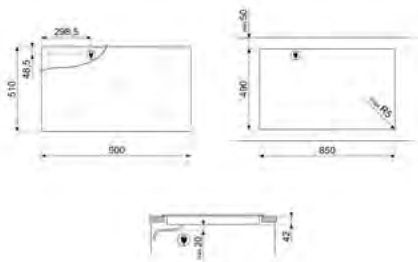
DESENHO TÉCNICO N° 32
