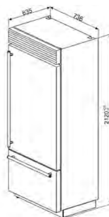
DESENHO TÉCNICO Nº 144
