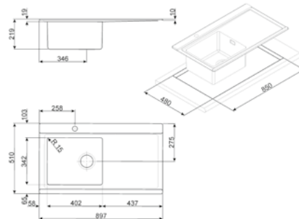
DESENHO TÉCNICO Nº 210
