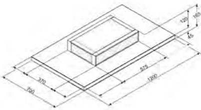
DESENHO TÉCNICO Nº 83
