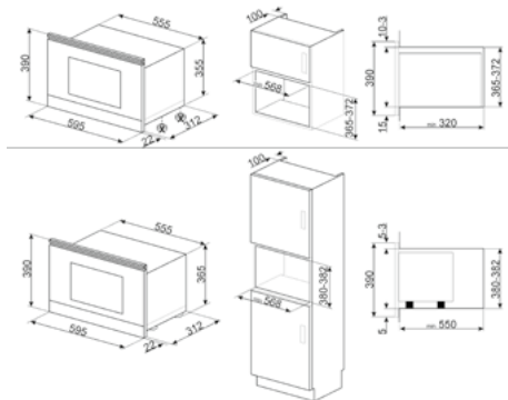
DESENHO TÉCNICO Nº 7
