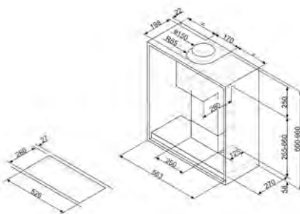
DESENHO TÉCNICO Nº 116
