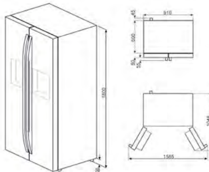
DESENHO TÉCNICO Nº 146
