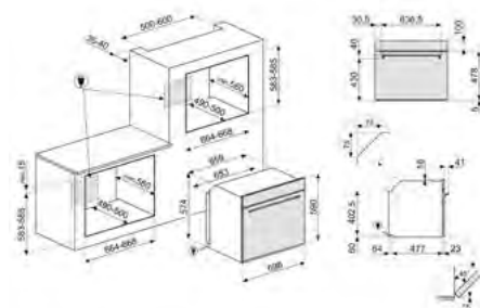
DESENHO TÉCNICO Nº 3
