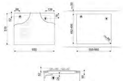
DESENHO TÉCNICO Nº 19
