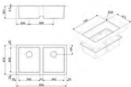
DESENHO TÉCNICO Nº 198
